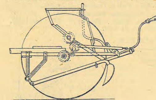
Sección longitudinal de la distribuidora Bousset
