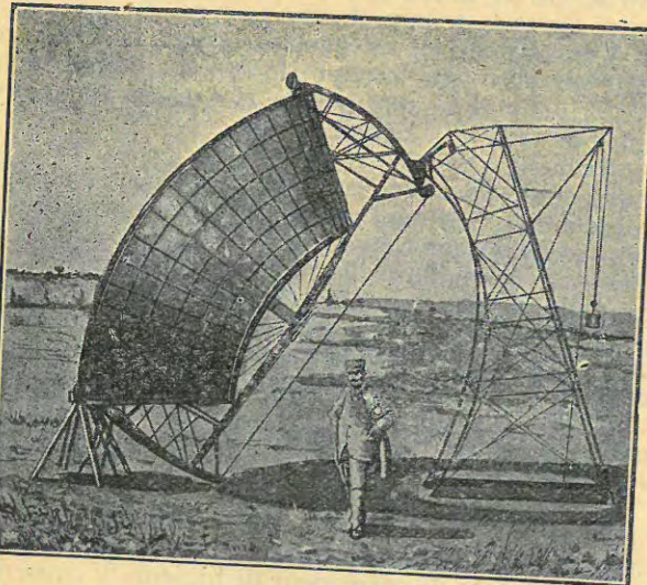
Motor solar visto de perfil
